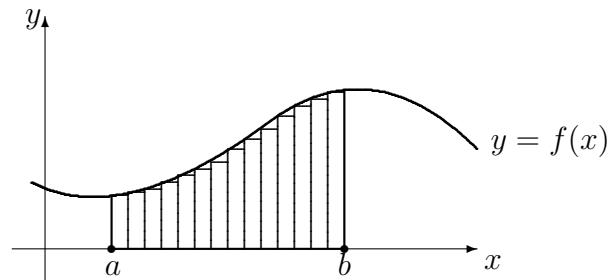
FIGURE 2.12 – Aire sous la courbe y = f(x) entre a et b ; somme à gauche avec 14 subdivisions.
