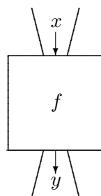
FIGURE 4.1 – Représentation d’une fonction.
